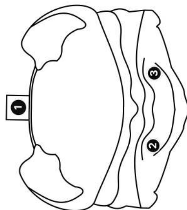
Thorax
