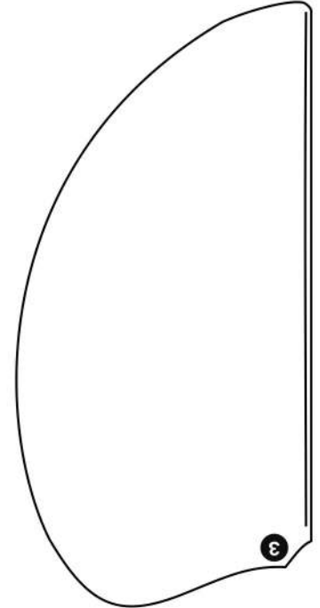
Elytron 2
